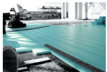
Protecção térmica do pavimento de um hangar de aviões com FIBRANxps
